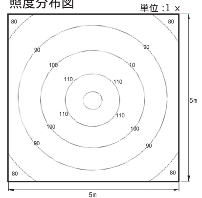
照度分布図
